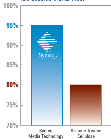
Separación de Agua Emulsionada (De acuerdo a SAE 1488)
