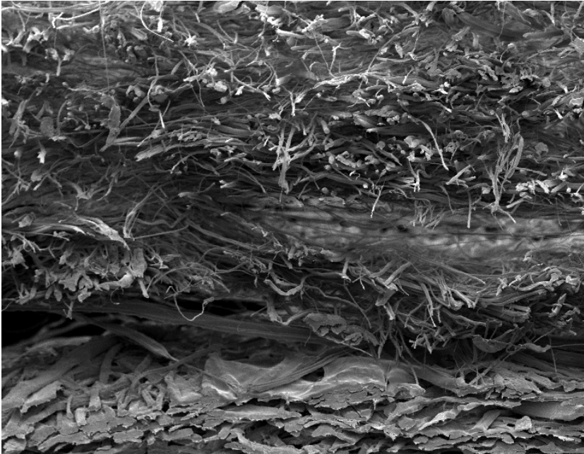
Medio filtrante para combustible Donaldson Synteq™ ampliado 100X
